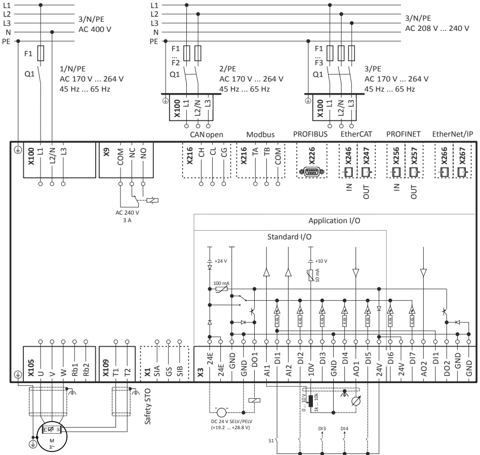
Fig. 2: Wiring example
